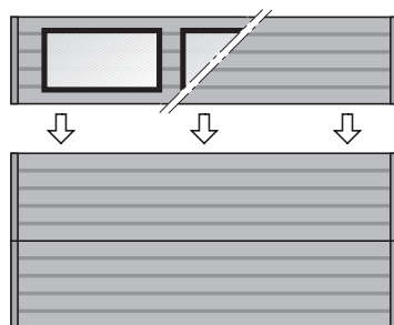
Porttype LDI: Isolerede sektioner
